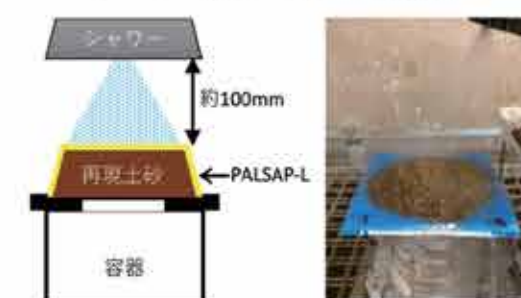
PALSAP-L散布後 78mm/h相当の雨でも破損無し
