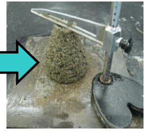
TG ブロック- \alpha 濃度 : 0.8% 注入率 : 30% ミスラン o 値 : 4.2 cm
