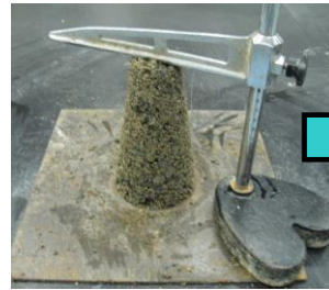
加泥材添加前性状 礫 50%、川砂 50%、 加水 5% ミスラン o 値 : 0 cm
