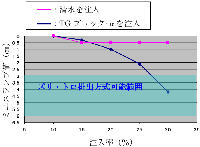
加泥材添加前性状 礫 50%、川砂 50%、 加水 5% ミスラン o 値 : 0 cm
